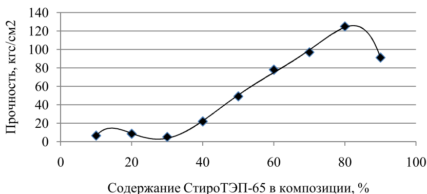
Рисунок – Влияние состава композиции СтироТЭП-65 - полигексен на когезионную прочность при разрыве
