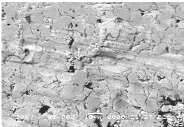
Рис. 6. Изношенные поверхности при упрочнении комплексным борированием зубчатых колес после 1,8 \times 10^7 циклов нагружения ( \times 1000 )
