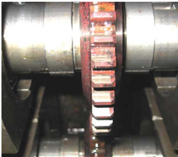
Рис. 3. Смещение зубчатых колес при проведении сравнительных испытаний
