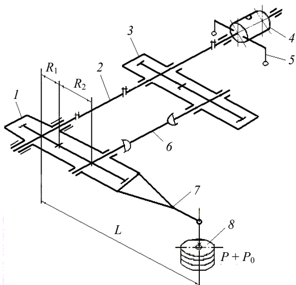
Рис. 1. Схема стенда для испытания зубчатых колес: 1 и 3 – редукторы с испытываемыми зубчатыми колесами; 2 и 6 – соединительные валы; 4 – электродвигатель; 5 – устройство измерения КПД стенда; 7 – рычаг; 8 – груз
