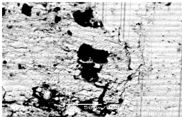
Рис. 4. Изношенные поверхности цементованных зубчатых колес после 1,8 \times 10^7 циклов нагружения при моменте M = 100 Нм ( \times 500 )
