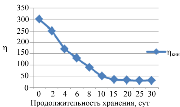
Изменение кинематической вязкости полиамидокислотных растворов в ДМФА в зависимости от продолжительности хранения при 20°C
