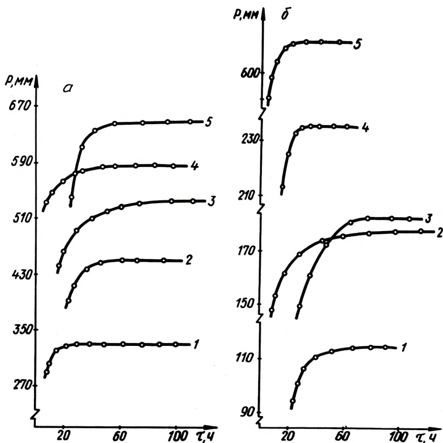
Рис. 1. Изотермические кривые, характеризующие установление равновесного давления водяных паров при изучении дегидратации кристаллогидратов тензиметрическим методом: а - \text{Mn}_3(\text{PO}_4)_2 \cdot 6\text{H}_2\text{O} (1); \text{Zn}_3(\text{PO}_4)_2 \cdot 4\text{H}_2\text{O} (2);
