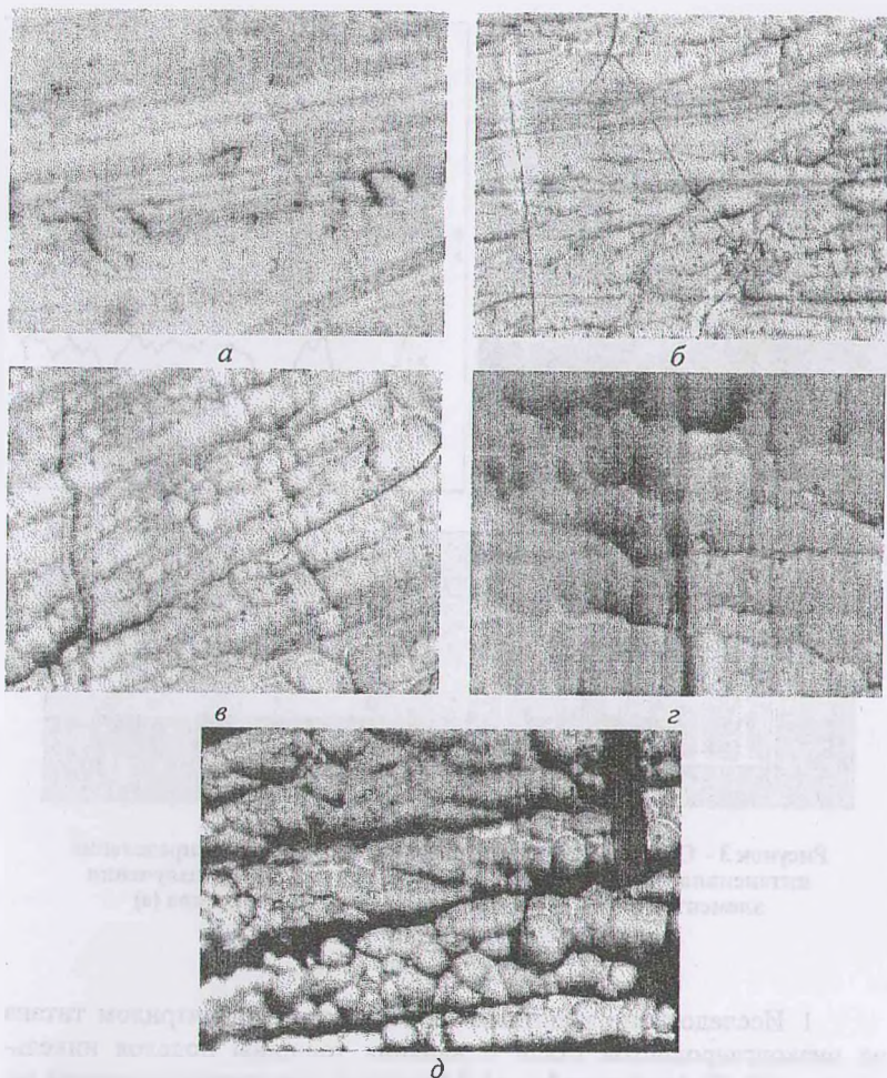
Рисунок 2 – Оптические снимки поверхности сплава, полученного при плотностях тока 2 \text{ A/dm}^2 (а), 4 \text{ A/dm}^2 (б), 5 \text{ A/dm}^2 (в), 7 \text{ A/dm}^2 (з), 9 \text{ A/dm}^2 (д)
