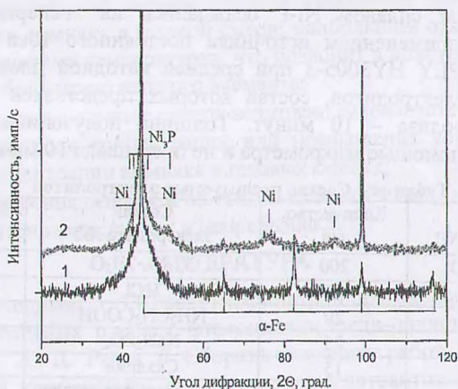
Рисунок 1 – Рентгенограммы покрытий Ni-P, полученных при плотностях тока 9 \text{ А/дм}^2 (1) и 7 \text{ А/дм}^2 (2)
