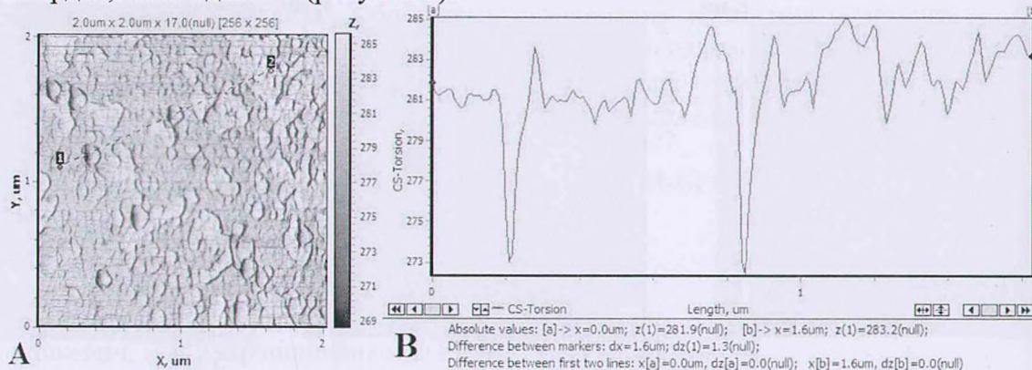
Рисунок 2. АСМ изображение в режиме «Torsion» (А) и профиль поперечного сечения (В) стекла, модифицированного ионно-ассистированным нанесением Мо с интегральным потоком ионов 8,1 \cdot 10^{16} ион/см 2
