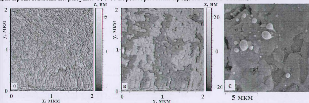
Рисунок 1. АСМ изображения топографии поверхности исходного стекла (А) и АСМ (В) и СЭМ (С) изображения поверхности стекла модифицированного ионно-ассистированным нанесением Mo с интегральным потоком ионов 1,2 \cdot 10^{16}
