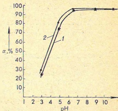
Рис. 1. Изменение степени осаждения P_2O_5 ( \alpha ) в зависимости от pH растворов:
