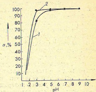
Рис. 2. Степень перехода фтора в осадок \alpha в зависимости от pH:
