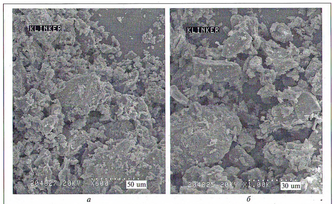
Микроструктура доломитового клинкера: а — температура обжига 1450 °С, время выдержки 30 мин; б — температура обжига 1500 °С, время выдержки 30 мин
