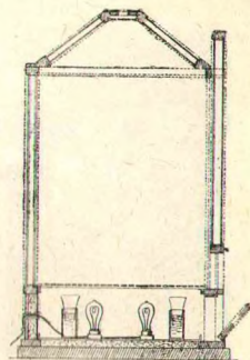
РАЗРЕЗ ПО АВ
