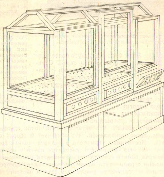
Рис. 2. Рабочий чертеж полигигростата. Деревянный каркас аппарата. Дверца камеры 2 приподнята; дверца нижнего помещения камеры 3 откинута. У подставки видна спереди выдвигающая доска, на которую ставятся приборы и сосуды во время наблюдений или очистки камеры.
