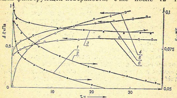
Рис. 3. Зависимость сопротивления фильтра \Delta P и скорости фильтрации v_{\text{ф}} от времени \tau :
