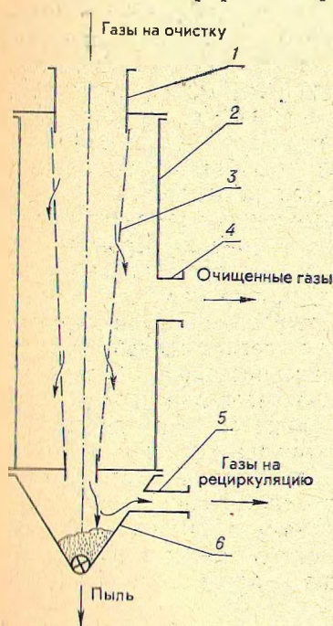
Рис. 1. Фильтр с конусным рукавом.
