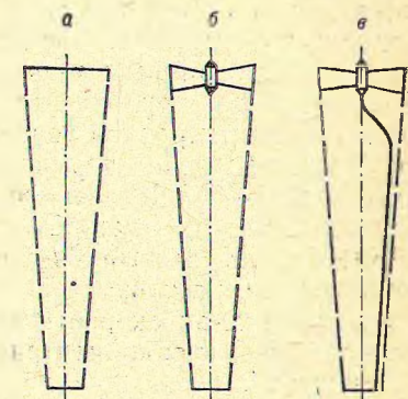
Рис. 2. Фильтрующие элементы конусной формы:
