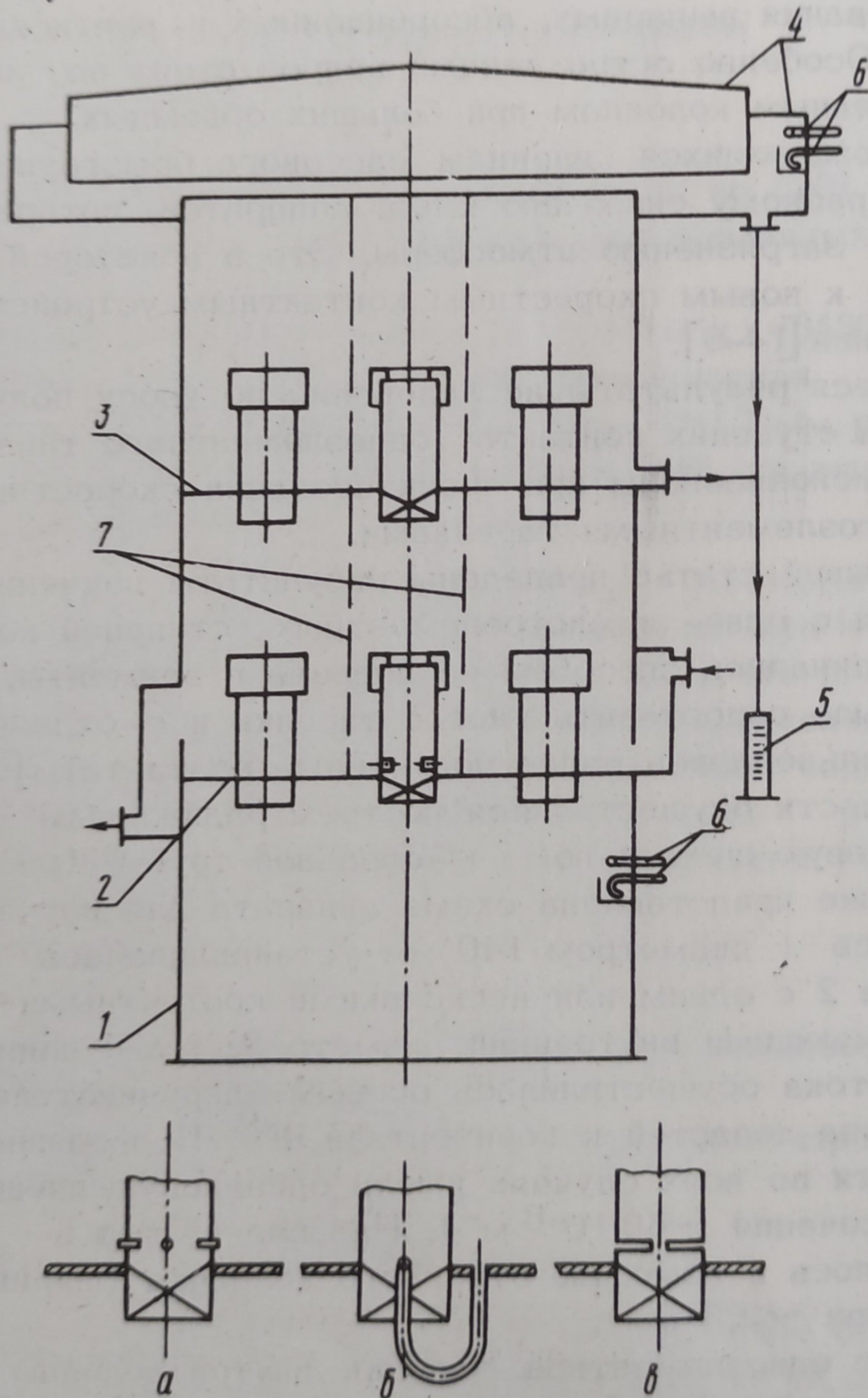
Рис. 1. Схема опытной колонны: а — радиальные трубки; б — U-образные трубки; в — кольцевая щель.
