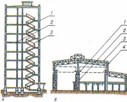
Будаўнічыя канструкцыі: а — буйнапанельнага жыллага дома (1 — сценавая панэль, 2 — панэль перакрыцця, 3 — лесвічны марш); б — прамысловага будынка (1 — падкранавая бэлька, 2 — калона, 3 — ферма перакрыцця, 4 — сценавая агароджа).
