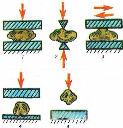
Спосабы драблення: 1 — расцісканне; 2 — расколванне; 3 — сціранне; 4, 5 — удары.
