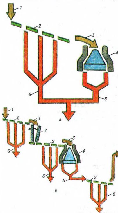
Схемы драблення: а — аднаступеньчаты цыкл; б — многаступеньчаты цыкл; 1 — матэрыял; 2 — грохат; 3 — буйныя фракцыі пасля грохата; 4 — конусная драблілька; 5 — фракцыі пасля драблення; 6 — дробныя фракцыі, адсартаваныя грохатам; 7 — шчокавая драблілька.
