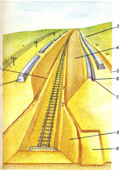
Земляное палатно чыгункі: 1 — кавальер; 2 — кювет; 3 — паласа адводу; 4 — выемка; 5 — нагорная канава; 6 — забанкетная канава; 7 — банкет; 8 — насып; 9 — рэзерв.
