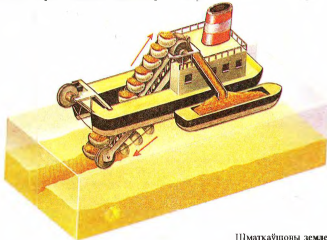
Шматкаўшова землярыйная машына.
