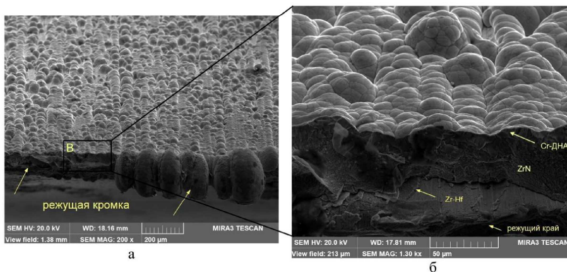
Рис. 1. СЭМ-снимки лезвия ножа с Cr-ДНА/ Hf – Zr – ZrN покрытием: (а) режущей кромки и (б) выделенной зоны В скола на острие лезвия
