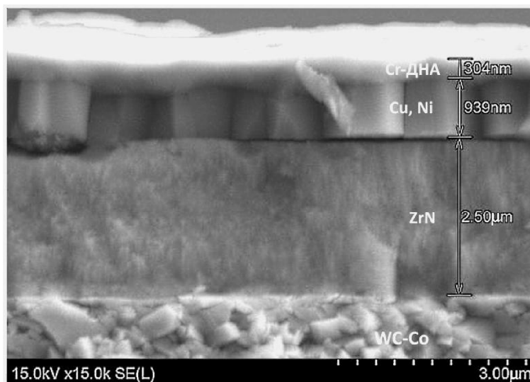
Рис. 2. Микроструктура Cr-ДНА/ ZrN покрытия на твердосплавной (WC – Co) основе
