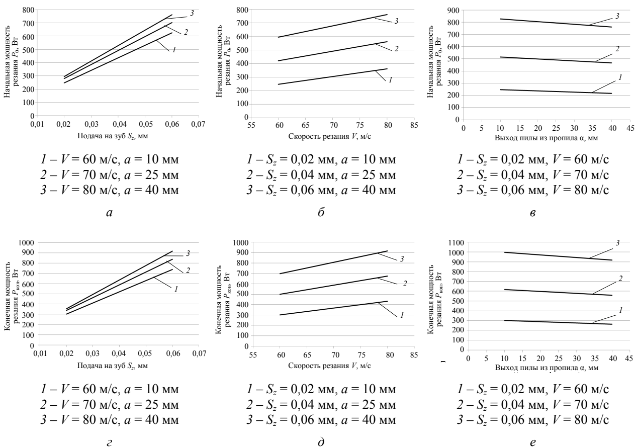
Рис. 2. Зависимости начальной ( а, б, в ) и конечной ( г, д, е ) полезной мощностей резания от переменных технологических факторов ( S_z, V, a ) при обработке ЛДСтП дисковыми твердосплавными пилами с плоско-треугольным с вогнутой передней гранью профилем зубьев
