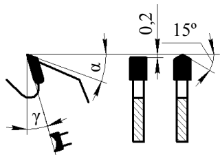
Рис. 1. Плоско-треугольный профиль зубьев с вогнутой передней гранью
