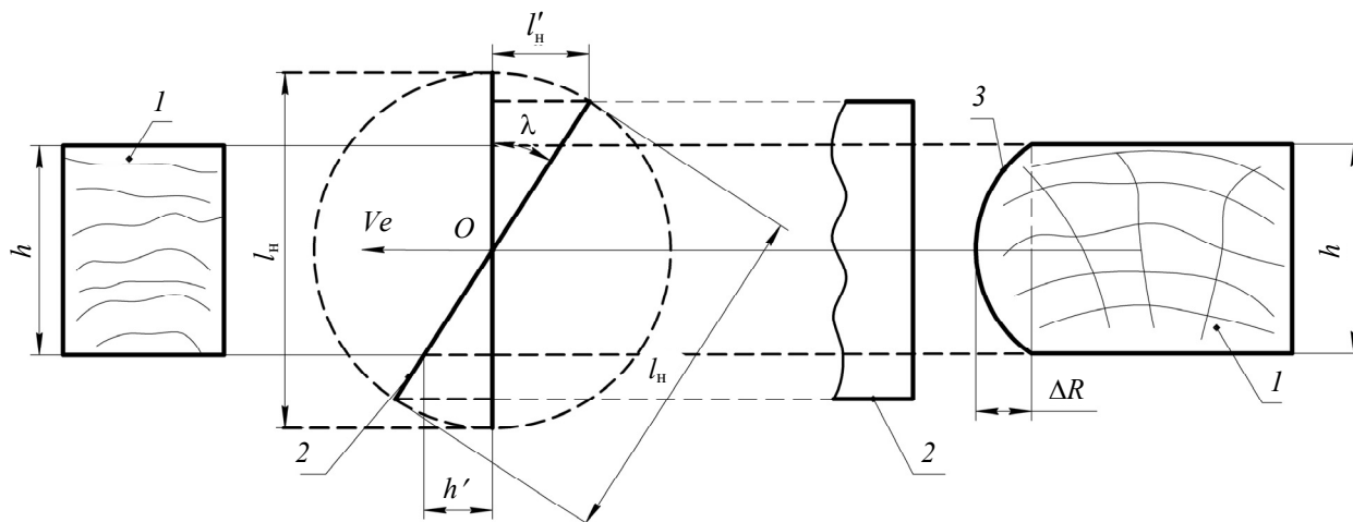
Рис. 3. Схема для расчета отклонения от плоскостности:
