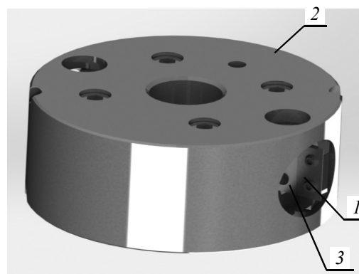
Рис. 1. Фреза сборная с изменяемыми углами передним и наклона кромки
