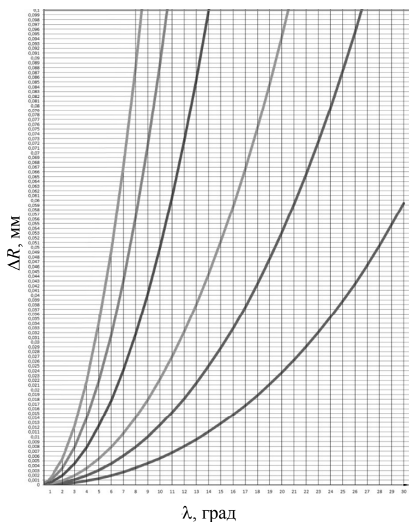
Рис. 5. Влияние угла наклона режущей кромки \lambda на величину отклонения от плоскостности \Delta R для установленных высот обрабатываемых деталей при фрезеровании режущей кромкой длиной l_{\text{н}} = 60 мм
