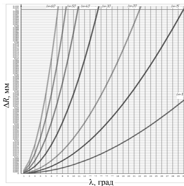
Рис. 4. Влияние угла наклона режущей кромки \lambda на величину отклонения от плоскостности \Delta R для установленных длин режущих кромок
