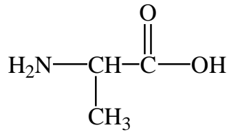
аланин
