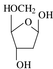
дезоксирибоза
