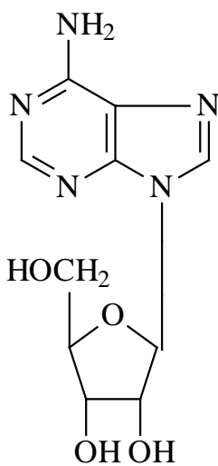
аденозин
