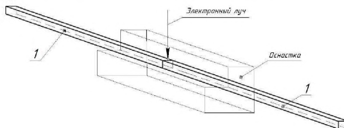
Рисунок 1 – Схема сварки ЭЛС: 1 – свариваемые образцы
