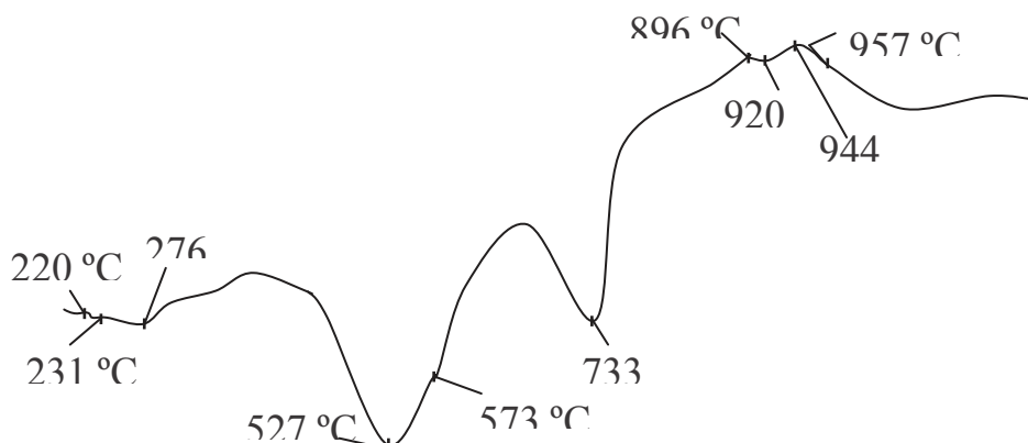
Рисунок – ДСК ангобного покрытия оптимального состава серии 2
