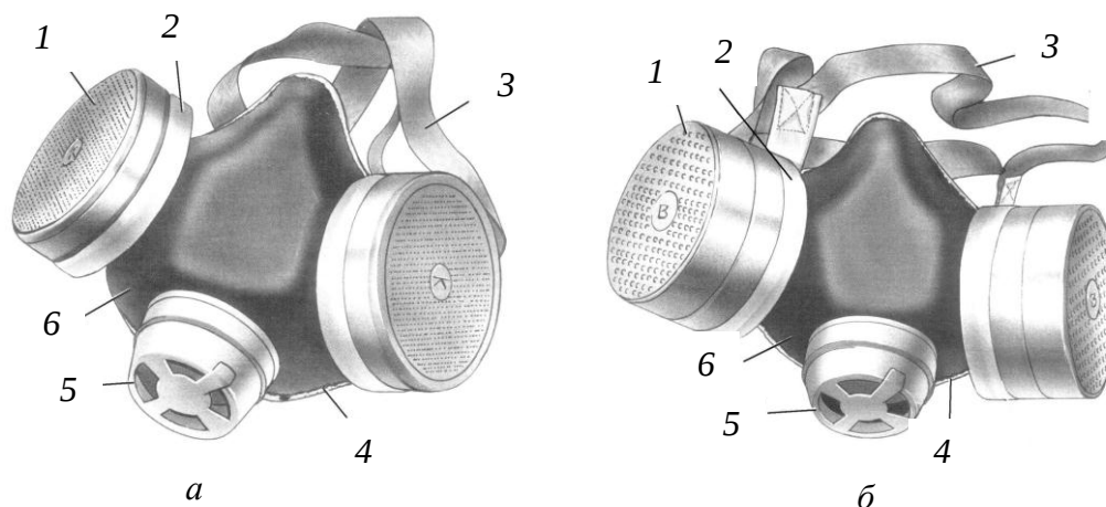
Рис. 23. Респираторы РПГ-67 (а), РУ-60М (б):
