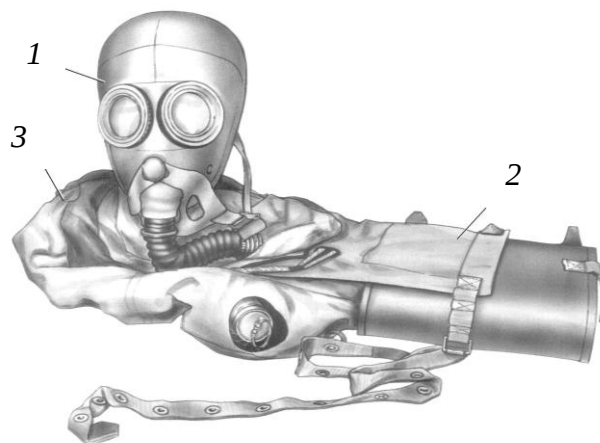
Рис. 25. Противогаз изолирующий ИП-5:
