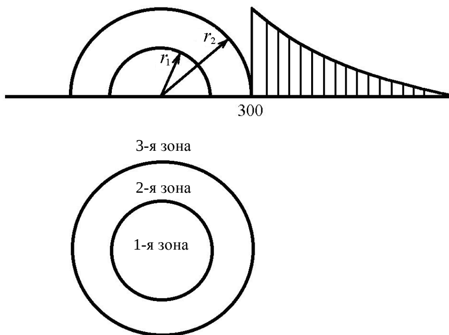
Рис. 2. Схема взрыва газовойздушной смеси
