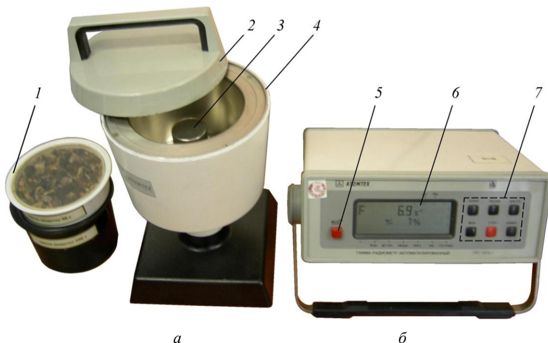
Рис. 7. Общий вид гамма-радиометра автоматизированного РКГ-02А/1: а – блок детектирования (БД): 1 – сосуд Маринелли с пробой; 2 – съемная крышка БД; 3 – сцинтиллятор NaI(Tl); 4 – свинцовая защита; б – блок обработки информации: 5 – кнопка включения прибора; 6 – экран индикатора; 7 – блок кнопок управления прибором
