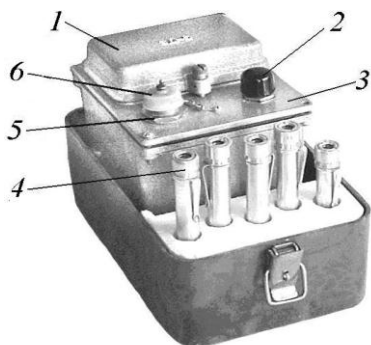
Рис. 10. Индивидуальный дозиметр ДП-24: 1 – крышка отсека питания; 2 – ручка потенциометра; 3 – зарядное устройство; 4 – дозиметр; 5 – зарядное гнездо; 6 – колпачок
