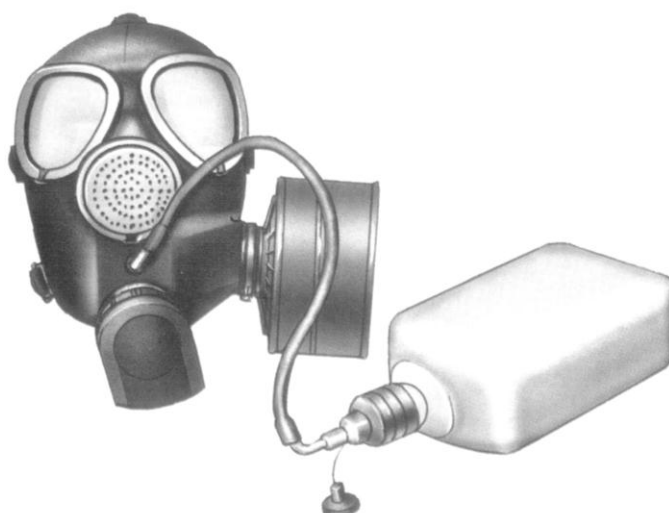
Рис. 17. Гражданский противогаз ГП-7ВМ
