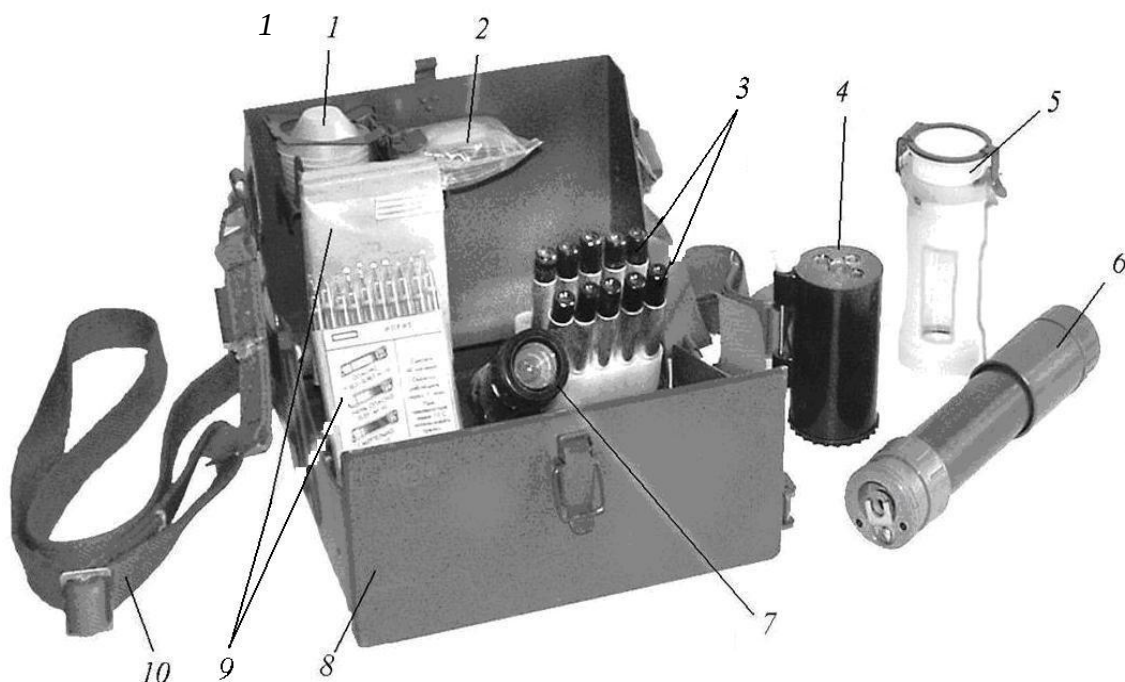
Рис. 13. Войсковой прибор химической разведки ВПХР:
