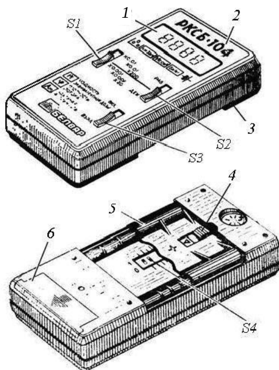
Рис. 5. Общий вид радиометра РКСБ-104:
