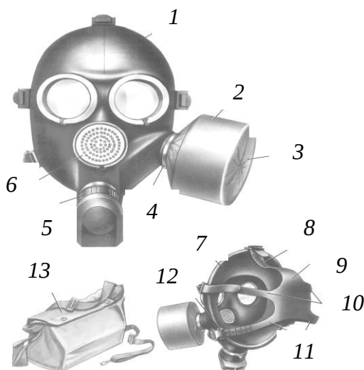
Рис. 15. Гражданский противогаз ГП-7: 1 – лицевая часть; 2 – фильтрующе-поглощающая коробка; 3 – трикотажный чехол; 4 – узел клапана вдоха; 5 – переговорное устройство (мембрана); 6 – узел клапанов выдоха; 7 – обтюратор; 8 – наголовник; 9 – лобная лямка; 10 – височные лямки; 11 – щечные лямки; 12 – пряжки; 13 – сумка
