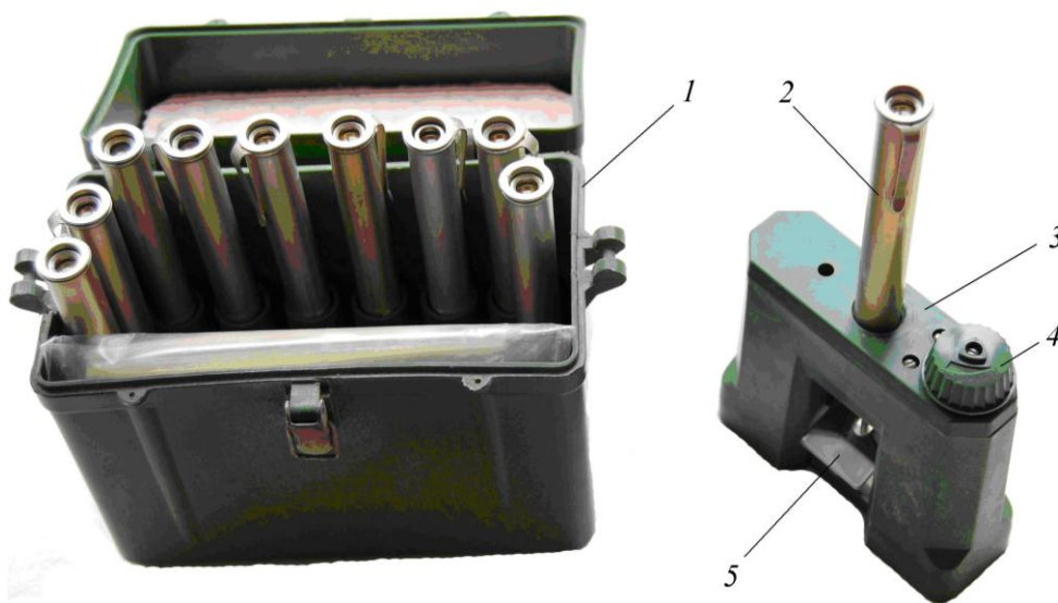
Рис. 11. Индивидуальный дозиметр ИД-1: 1 – футляр; 2 – измеритель дозы ИД-1; 3 – зарядное устройство ЗД-6; 4 – ручка зарядно-контактного узла; 5 – поворотное зеркало
