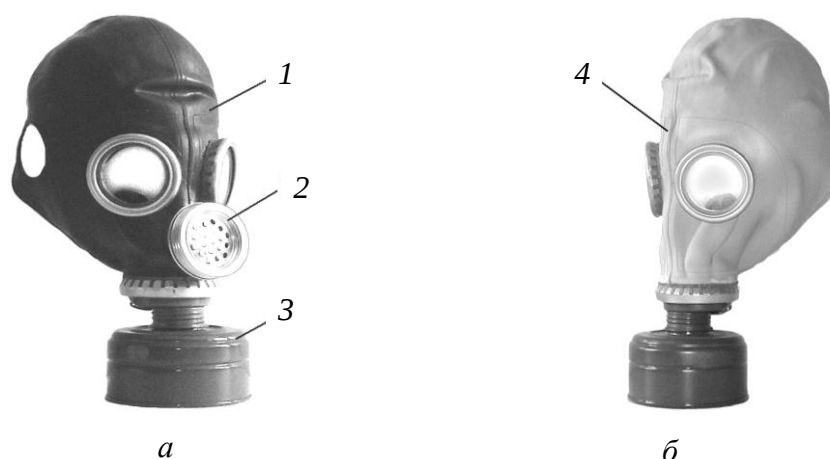
Рис. 14. Противогазы ГП-5М (а) и ГП-5 (б): 1 – шлем-маска ШМ-66МУ; 2 – переговорное устройство; 3 – фильтрующее-поглощающая коробка; 4 – шлем-маска ШМ-62У
