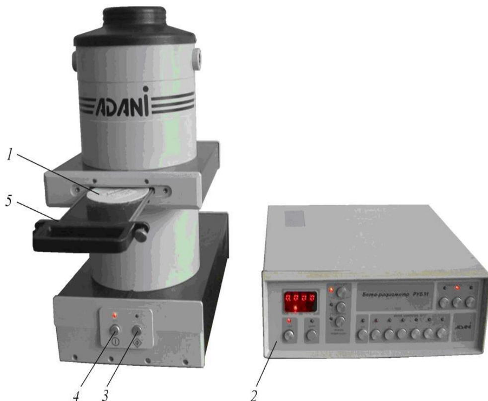
Рис. 8. Общий вид бета-радиометра РУБ-91 «АДАНИ»: 1 – исследуемый образец (проба); 2 – блок анализаторов; 3 – кнопка включения высоковольтных источников питания ФЭУ; 4 – кнопка включения и выключения прибора; 5 – предметный столик
