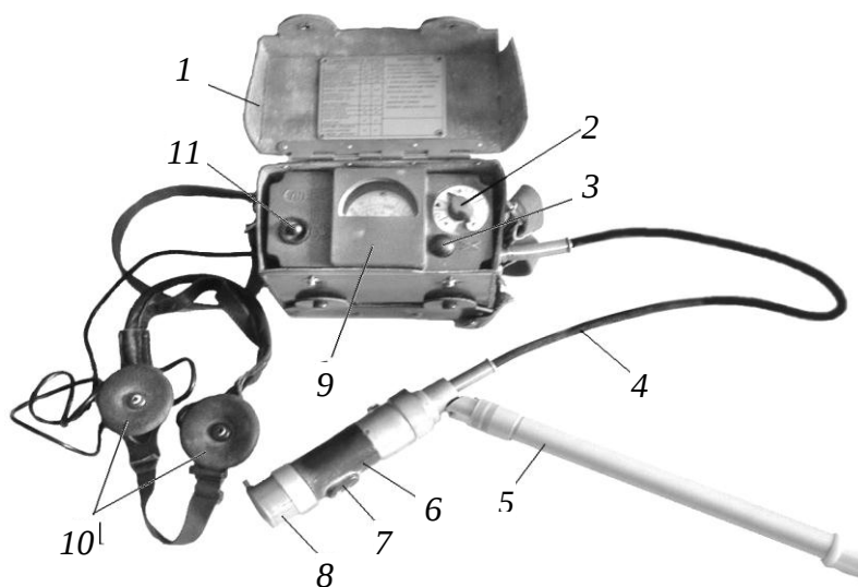
Рис. 4. Переносной измеритель мощности дозы ДП-5В:
