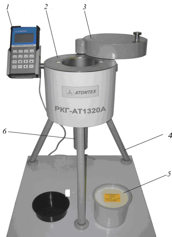
Рис. 9. Общий вид гамма-радиометра РКГ-АТ1320А: 1 – блок обработки информации с ЖКИ; 2 – блок защиты; 3 – крышка блока защиты; 4 – ножки с опорами; 5 – измерительный сосуд; 6 – блок детектирования
