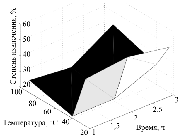
Рис. 7. Зависимость степени выщелачивания РЗЭ от температуры процесса и времени обработки
