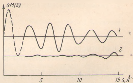
Экспериментальная функция интенсивности рассеяния электронов (1) и разность между наилучшей теоретической и экспериментальной кривыми (2)
