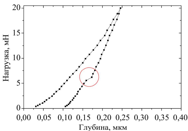
Рис. 3. Кривая нагрузки-разгрузки от образца кремния с покрытием на основе Mo
