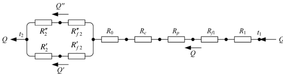
Рис. 4. Схема для расчета коэффициента теплопередачи
