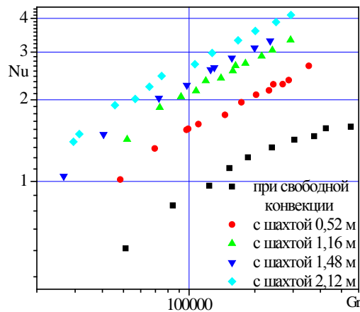
Рис. 3. Интенсификация теплоотдачи пучка воздействием вынужденной конвекцией
