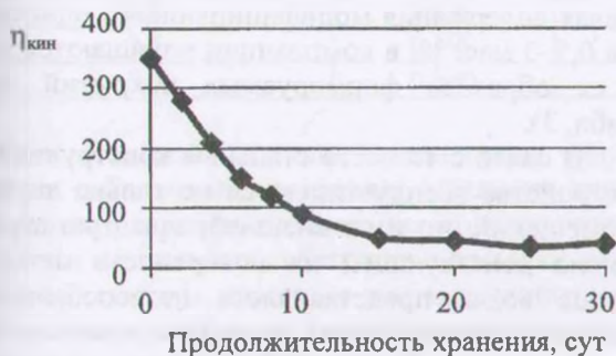
Рис. 1. Изменение кинематической вязкости полиимидных композиций в зависимости от продолжительности хранения при 20°C
