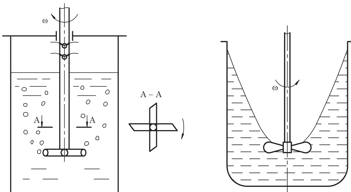
Рис. 6.6. Самовсасывающая мешалка
