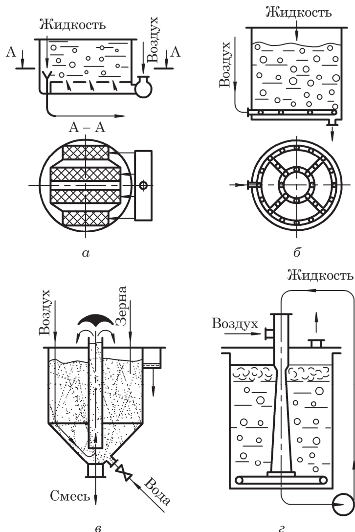
Рис. 6.15. Схемы пневматических (барботажных) перемешивающих устройств: а – с горизонтальной распределительной сеткой; б – с барботером; в – с эрлифтом; г – с сочетанием барботера и лопастной мешалки
