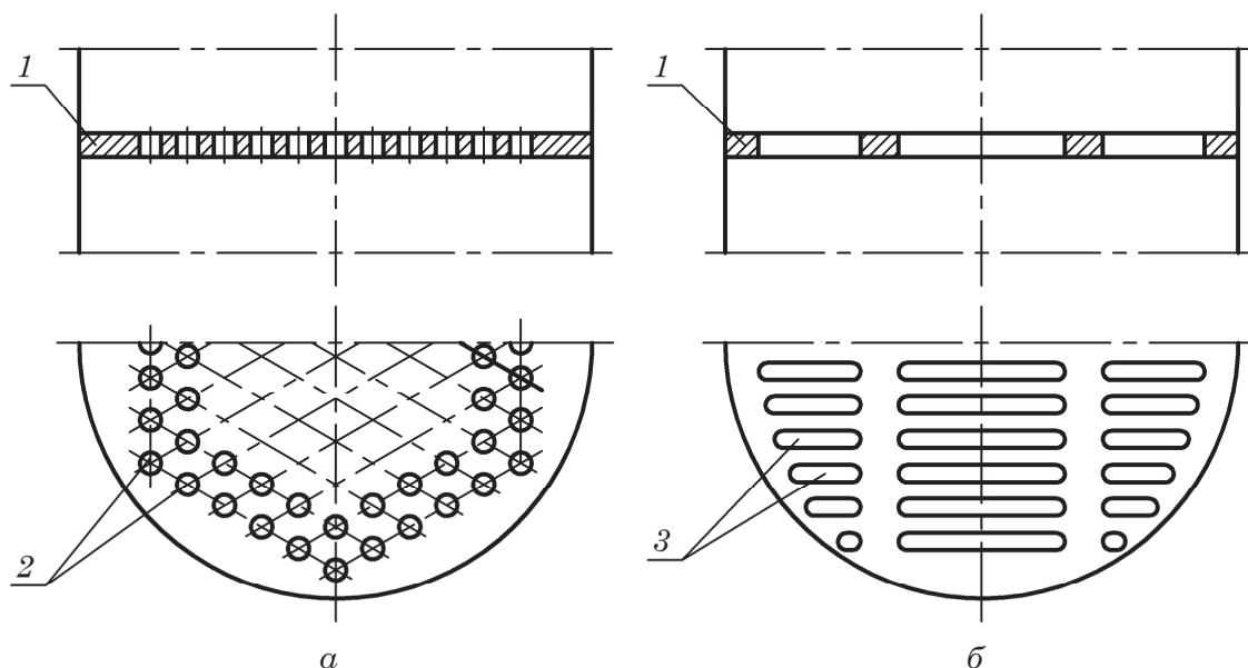
Рис. 5.24. Провальные тарелки: а – дырчатая; б – решетчатая; 1 – тарелка; 2 – отверстия; 3 – щели
