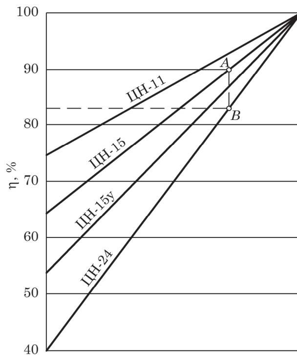
Рис. 7.9. Изменение коэффициента очистки газа \eta в зависимости от типа циклона
