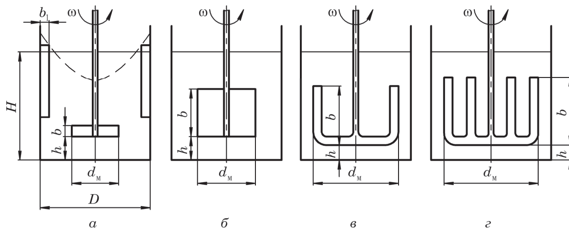
Рис. 6.2. Тихоходные мешалки:
