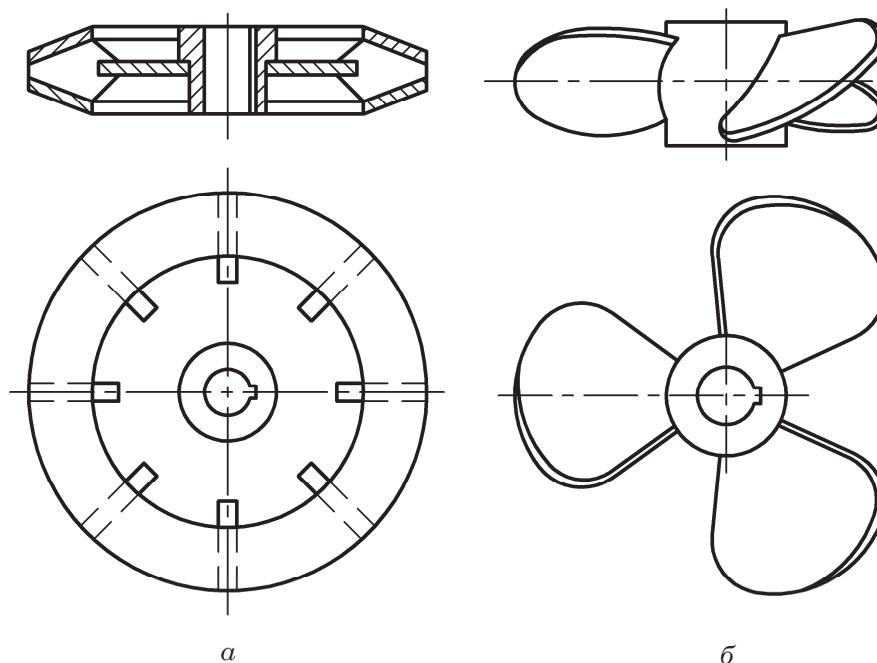
Рис. 6.3. Быстроходные мешалки:
