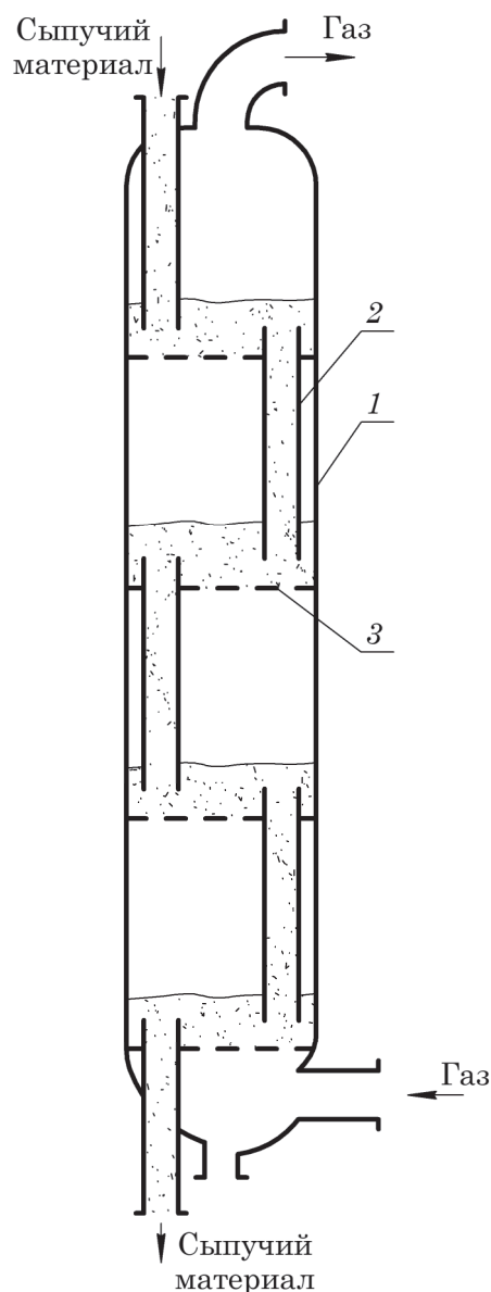
Рис. 5.7. Многоступенчатый адсорбер кипящего слоя: 1 – корпус; 2 – переточные трубы; 3 – перфорированные тарелки
