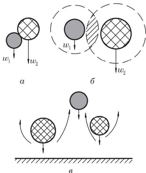
Рис. 2.8. Схема стесненного осаждения частиц различного диаметра
