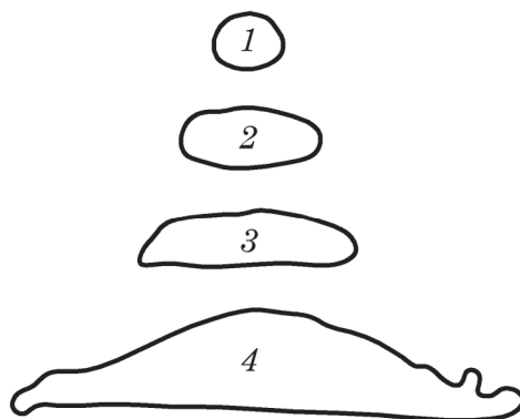
Рис. 5.15. Форма всплывающих пузырей: 1 – d < 1,5 мм; 2 – 1,5 < d < 5 мм; 3 – 5 < d < 25 мм; 4 – d > 25 мм
