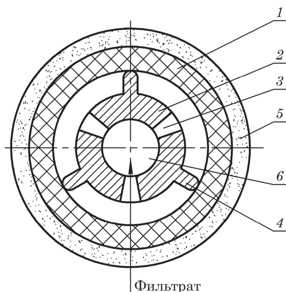
Рис. 3.10. Схема фильтровального патрона: 1 – пористые фильтровальные кольца; 2 – центральная труба; 3 – радиальное отверстие; 4 – продольные ребра; 5 – слой осадка; 6 – вертикальный канал
