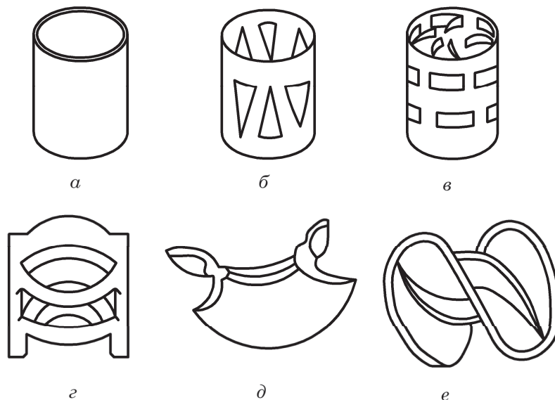
Рис. 5.29. Виды насадок: a – кольца Рашига; б – кольца Белецкого; в – кольца Палля; г – кольца Интерпак; д – седла Инталокс; е – седла Берля
