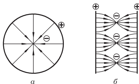
Рис. 7.24. Создание неоднородного электрического поля: а – в цилиндрической трубе; б – между параллельными пластинами
