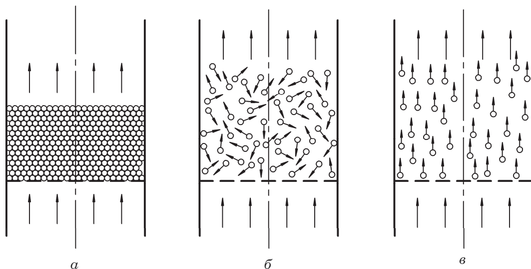
Рис. 5.1. Движение газа (жидкости) через слой зернистого материала: а – неподвижный слой; б – кипящий (псевдооживленный) слой; в – унос твердых частиц потоком
