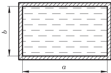
Рис. 1.4. К расчету эквивалентного диаметра прямоугольного поперечного сечения
