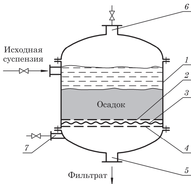
Рис. 3.5. Схема нутч-фильтра:
