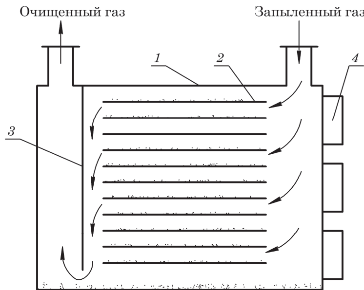
Рис. 2.12. Схема пылеосадительной камеры: 1 – корпус; 2 – полки; 3 – отражательная перегородка; 4 – люки для удаления пыли
