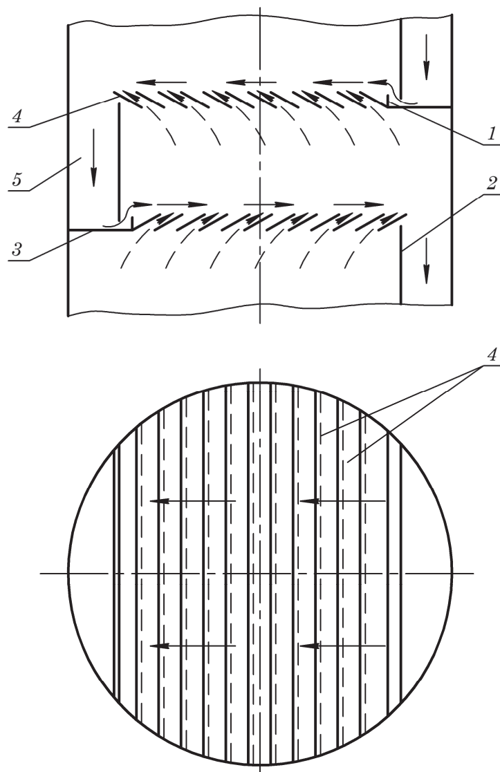
Рис. 5.23. Пластинчатая тарелка:
