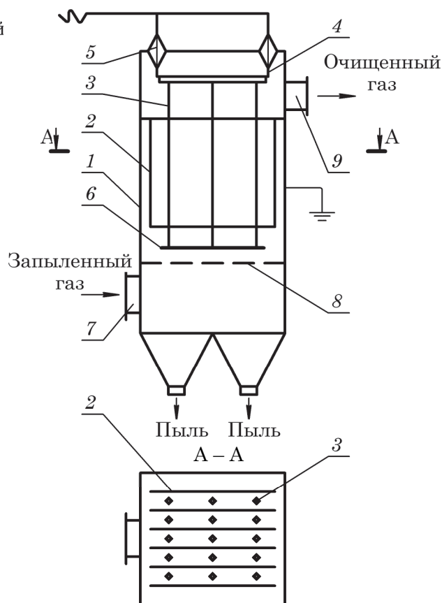
Рис. 7.26. Пластинчатый электрофильтр: 1 – камера; 2 – осадительный электрод; 3 – коронирующий электрод; 4 – рама; 5 – изолятор; 6 – рама; 7 – входной патрубок; 8 – распределительная решетка; 9 – выходной патрубок
