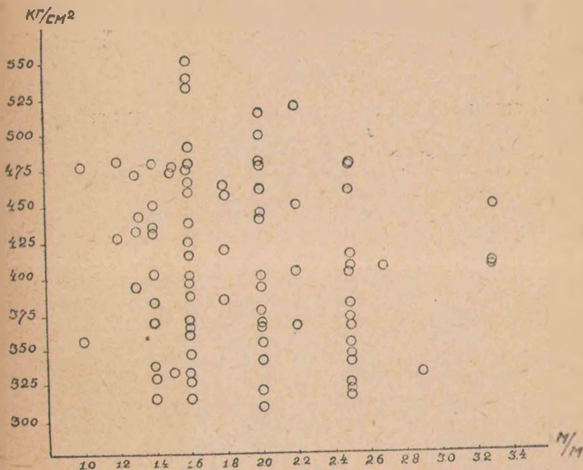
Зависимость между шириной годового слоя и временным сопротивлением сжатию вдоль волокон черного дуба
