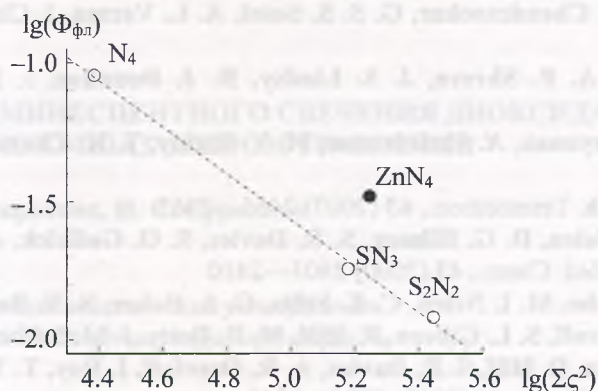
Рис. 5. Зависимость квантового выхода флуоресценции \Phi_{fl} исследуемых соединений от \Sigma\zeta^2 в двойных логарифмических координатах
