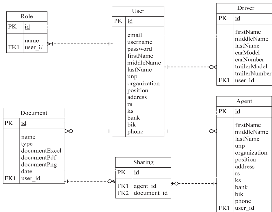
Рис. 3.4. Логическая схема данных
