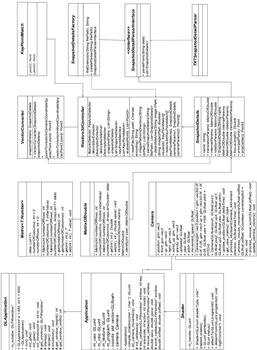
Рис. 3.3. Диаграмма классов
