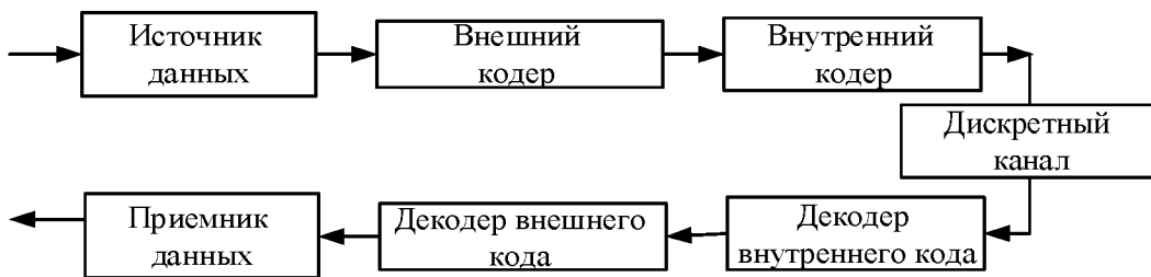
Рисунок 1 – Принципиальная схема последовательного каскадного кода с двумя компонентными кодами
