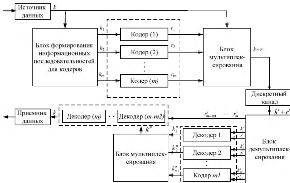
Рисунок 2 – Структурная схема последовательно-параллельной схемы кодирования с m компонентными кодами
