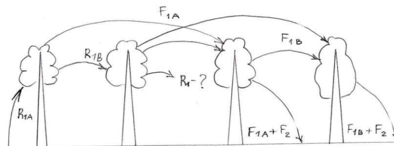
Рисунок 1 – Схема развития и заселения деревьев сосны вершинным короедом в течение вегетационного периода: R_{1A} – родительское поколение вершинного короеда, вышедшее из мест зимовки и заселившее дерево; R_{1B} – те же жуки, заселившие второе дерево; F_{1A} – молодые особи (первое поколение), заселяющие новые деревья; F_{1B} – те же жуки, заселившие второе дерево; F_2 – молодые особи второго поколения, уходящие на зимовку, или остающиеся зимовать в местах отрождения.
