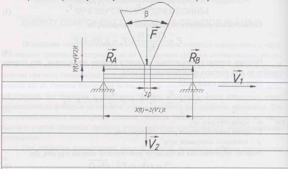
Рисунок 1 – Расчетная схема
