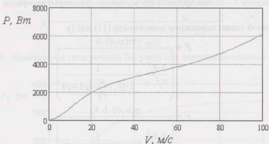
Рисунок 7 – Мощность резания с учетом сил инерции со стороны стружки
