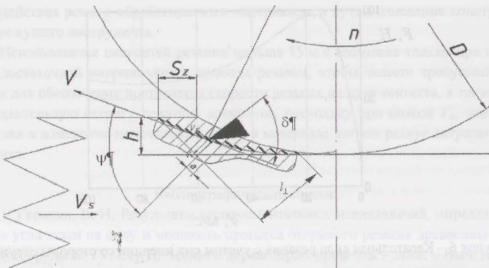
Рисунок 5 – Схема процесса фрезерования древесного материала
