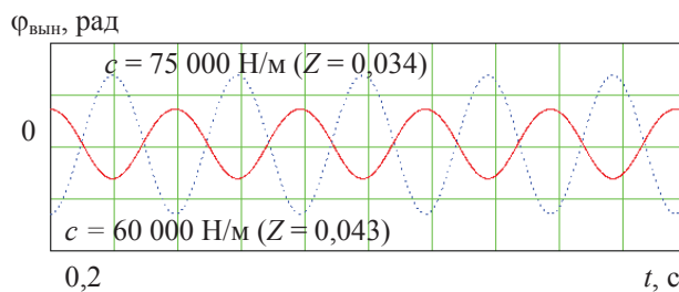
Рис. 6. Условия работы инструмента с самоизменяющимися углами резания
