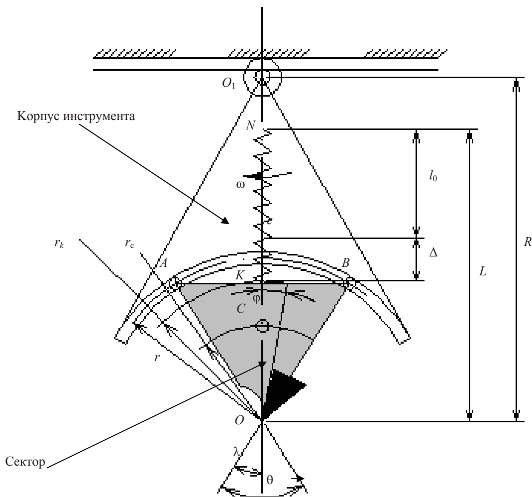
Рис. 1. Расчетная схема фрезерного инструмента с самоустанавливающимися углами резания
