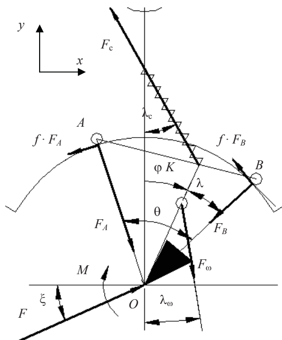
Рис. 3. Внешние силы, действующие на сектор инструмента
