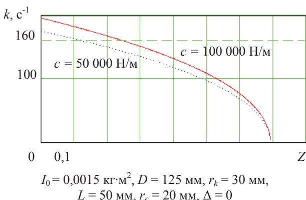
Рис. 5. Зависимость частоты собственных колебаний от частоты вращения инструмента
