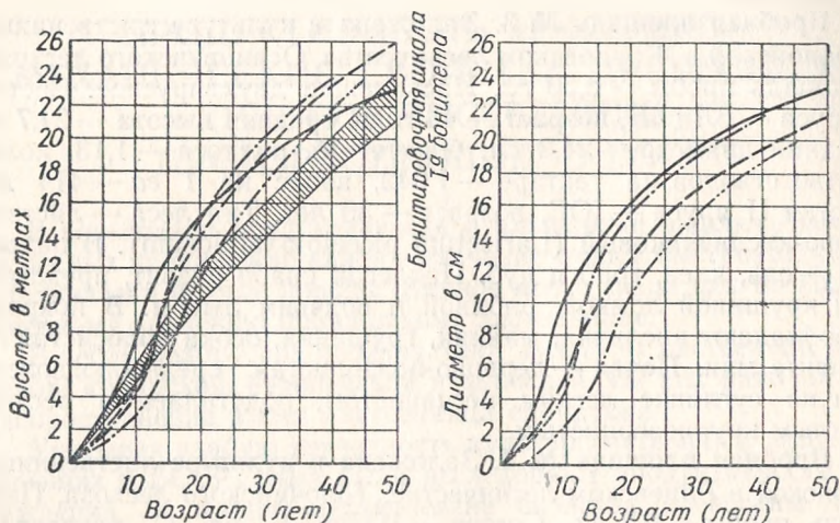
Рис. 1. Ход роста по высоте и диаметру культур лиственницы сибирской, лиственницы европейской и лиственницы японской. Условные обозначения:—лиственница сибирская
