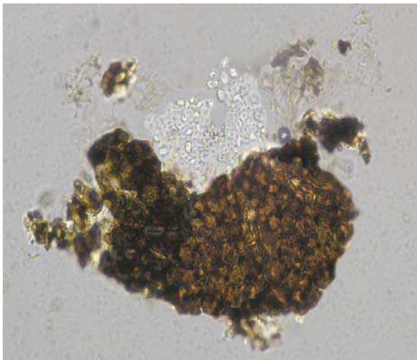
Рис. 1. Пикнида, конидиогенные клетки и споры Rhizosphaera kalkhoffii
