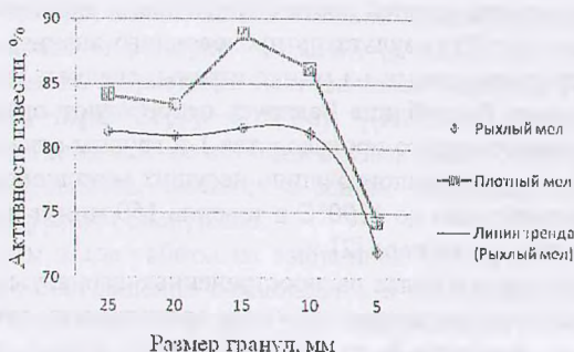
Рисунок 1 – Зависимость активности извести от фракционного состава мела
