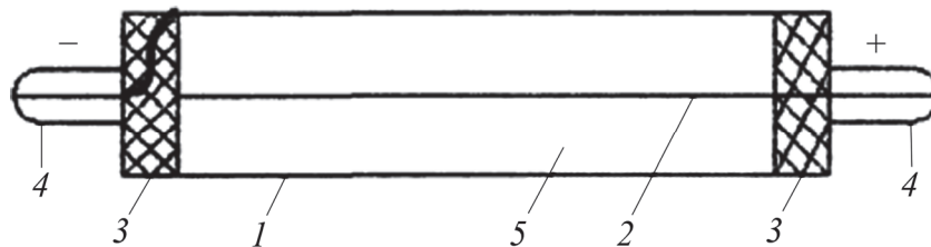
Рис. 6.4. Газоразрядный счетчик: 1 – металлический цилиндр (отрицательный электрод); 2 – тонкая металлическая нить (положительный электрод); 3 – изоляторы; 4 – выводные контакты; 5 – газовая среда, смесь инертных газов с галогенами при пониженном давлении
