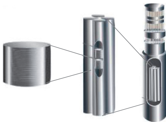
Рис. 3.10 Урановые таблетки в герметичной оболочке
