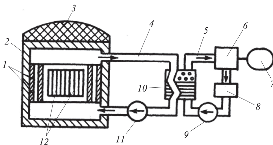
Рис. 3.8. Принципиальная схема АЭС ВВЭР-1000:
