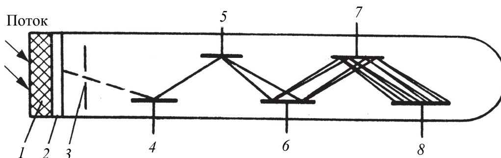
Рис. 6.6. Сцинтилляционный счетчик:
