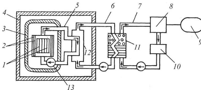
Рис. 3.9. Технологическая схема АЭС с реактором на быстрых нейтронах:
