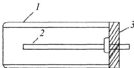
Рис. 6.1. Ионизационная камера: 1 – корпус; 2 – собирающий электрод; 3 – изолятор
