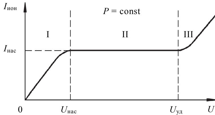
Рис. 6.3. Вольт-амперная характеристика ионизационной камеры: I – область рекомбинации; II – область насыщения; III – область ударной ионизации
