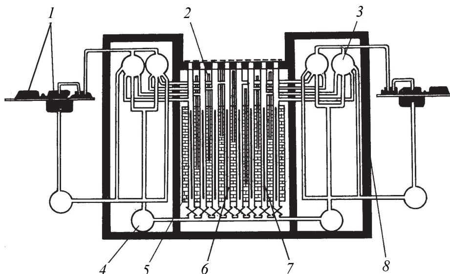
Рис. 3.7. Реактор большой мощности каналный на тепловых нейтронах РБМК-1000:
