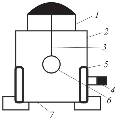
Рис. 6.5. Торцовый альфа-счетчик:
