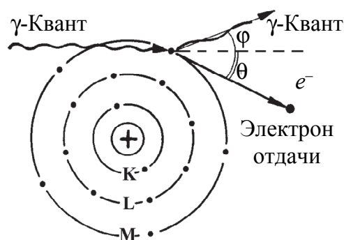
Рис. 4.5. Комптон-эффект
