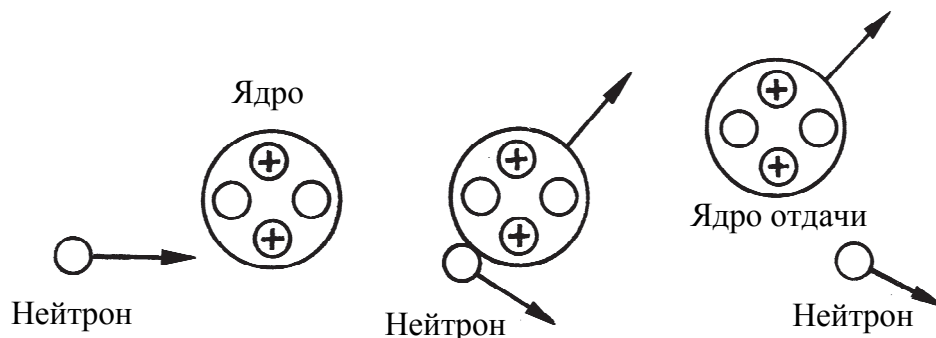
Рис. 4.1. Упругое столкновение нейтрона с ядром
