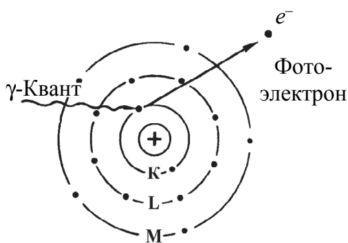
Рис. 4.4. Фотоэффект
