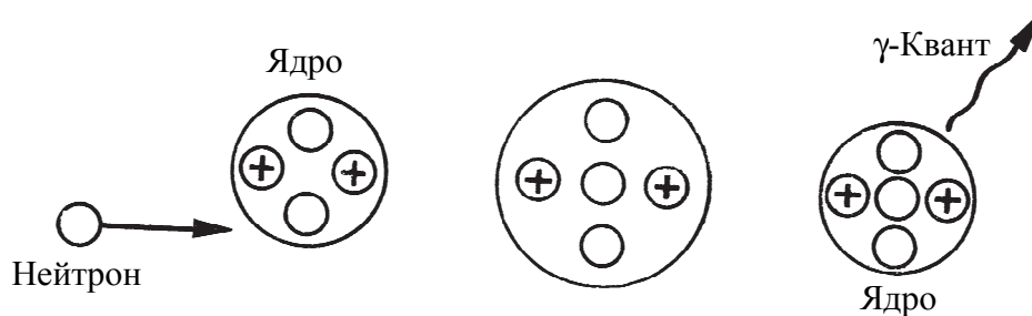
Рис. 4.3. Захват нейтрона ядром
