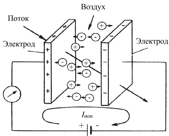
Рис. 6.2. Цепь ионизационной камеры
