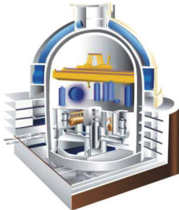
Рис. 3.11 Контейнмент
