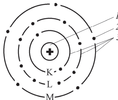
Рис. 3.2. Схема атомных электронных оболочек: 1 – ядро; 2 – электроны; 3 – электронные оболочки
