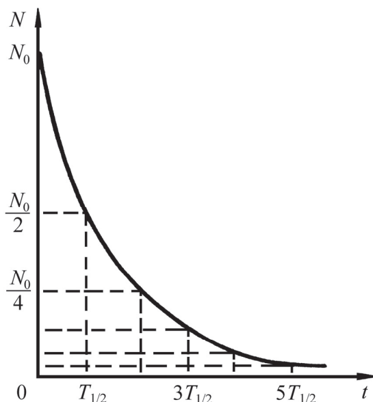
Рис. 3.4. График радиоактивного распада: N_0 – исходное количество радиоактивного вещества; T_{1/2} – период полураспада вещества
