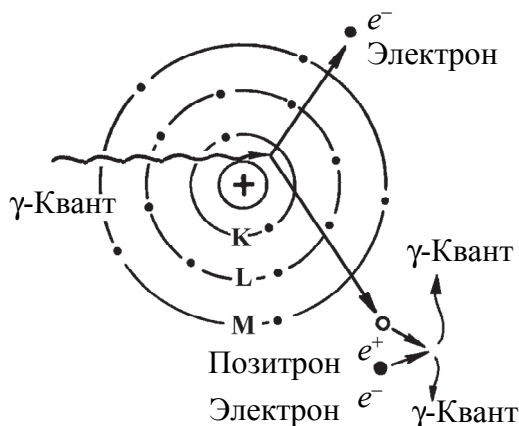
Рис. 4.6. Образование электронно-позитронной пары
