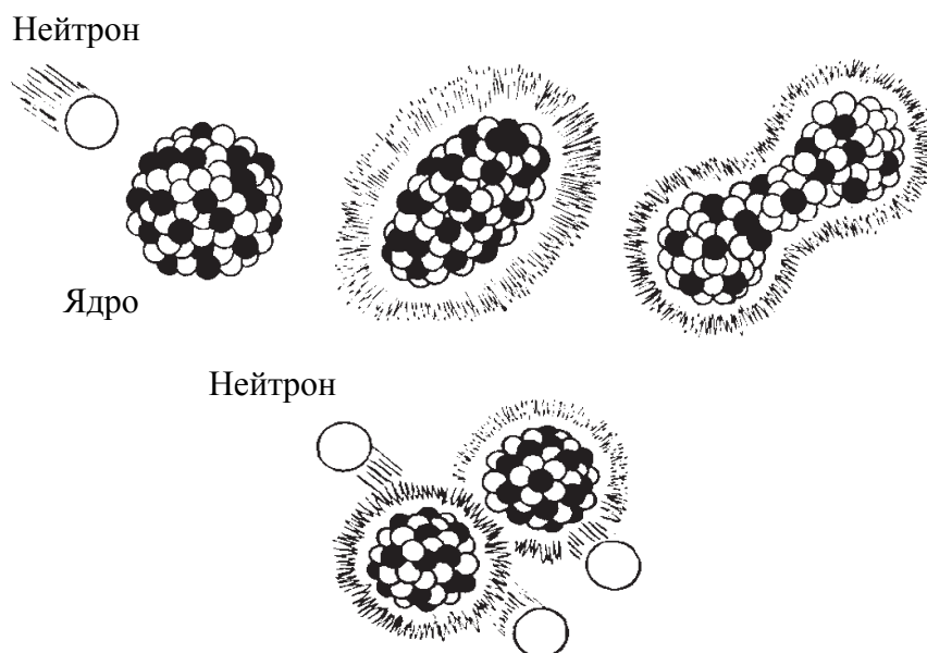
Рис. 3.5. Механизм деления тяжелых ядер
