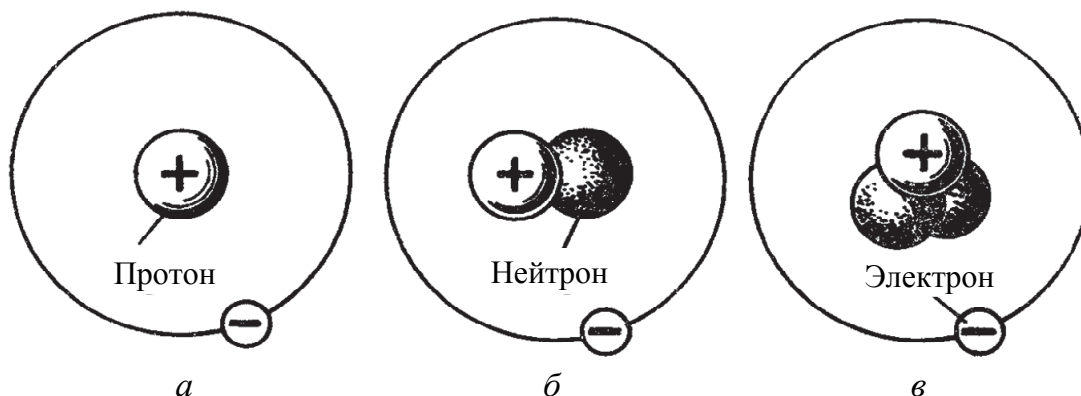
Рис. 3.3 Схема строения атомов изотопов водорода: a – водород; b – дейтерий; v – тритий
