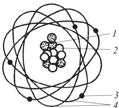
Рис. 3.1. Строение атома: 1 – протон; 2 – нейтрон; 3 – электрон; 4 – орбиты
