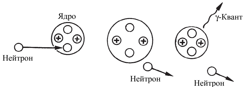
Рис. 4.2. Неупругое столкновение нейтрона с ядром
