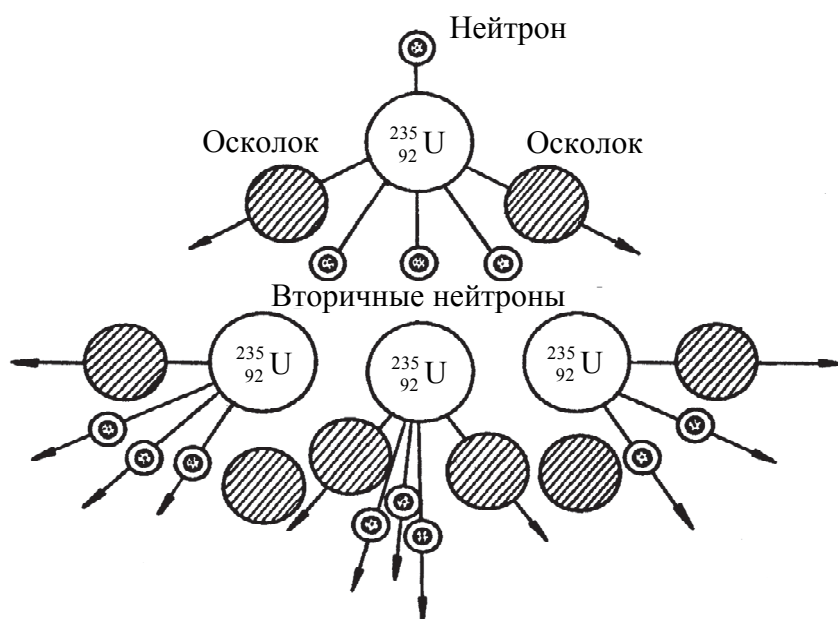
Рис. 3.6. Цепная ядерная реакция деления ^{235}_{92}\text{U}
