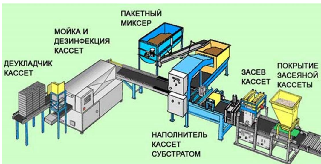
Рисунок 5. Схема технологической линии для посева кассет
