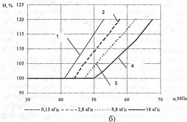
Рис. 1. Пороговые напряжения стали 40Х (а) и стали 10 (б) определенные на различных частотах испытаний.
