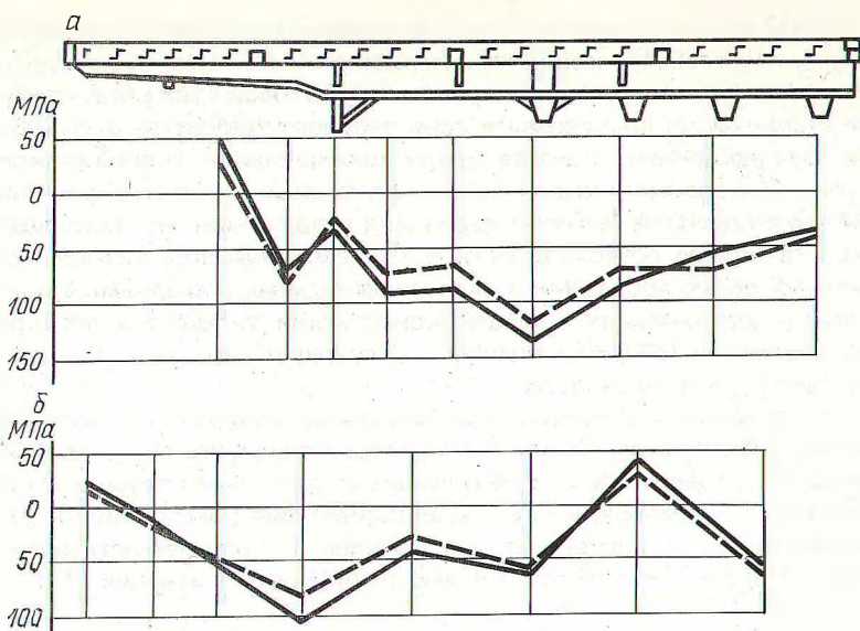
Рис. 1. Суммарные напряжения на краю нижних полок лонжерона и боковой балки при движении со скоростью 35 км/ч по гравийному (сплошные линии) и булыжному (штриховые) покрытию: а — лонжерон; б — боковая балка.
