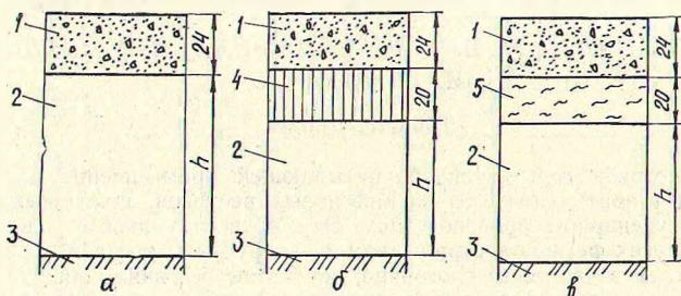
Конструкции дорожных одежд опытных участков: а — участок № 1 (контрольный); б — участок № 2; в — участок № 3; 1 — дорожная одежда; 2 — земляное полотно; 3 — основание земляного полотна; 4 — гидролизный лигнин; 5 — древесные опилки; h — высота земляного полотна
