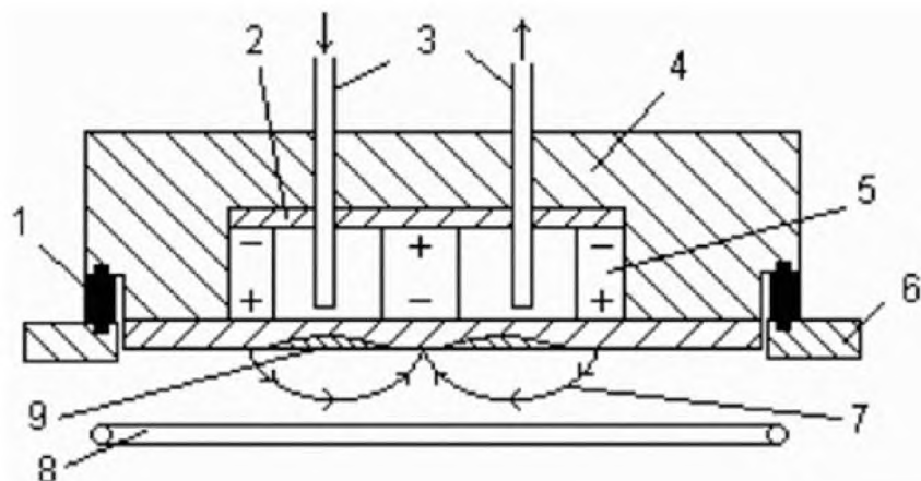
1 – изолятор; 2 – магнитопровод; 3 – система водоохлаждения; 4 – корпус катодного узла; 5 – постоянный магнит; 6 – стенка вакуумной камеры; 7 – силовые линии магнитного поля; 8 – кольцевой водоохлаждаемый анод; 9 – зона эрозии распыляемого катода
