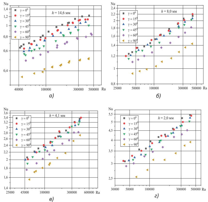
Рис. 1. Свободно-конвективная теплоотдача ребристых труб при углах наклона \gamma = 0, 15, 30, 45, 60 и 90^\circ к горизонтальной плоскости с различными высотами ребра труб:
