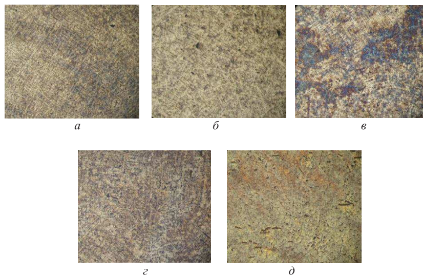
Рисунок 1 – Дендриты первичного аустенита немодифицированного ( а ) и модифицированного FeSiBa ( б ), модифицированного FeSiBa + лигатура ( в ), модифицированного FeSiBa + выд. 15 мин ( г ), модифицированного FeSiBa + лигатура + выд. 15 мин ( д ) серого чугуна ( \times 50 )
