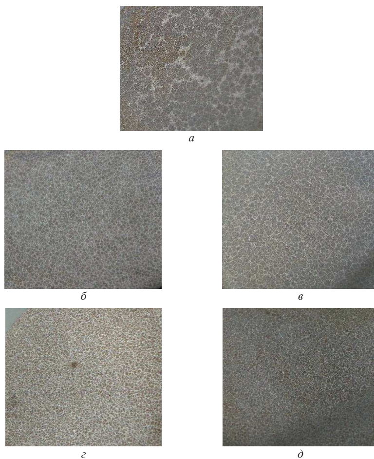
Рисунок 2 – Эвтектические зерна немодифицированного ( a ) и модифицированного FeSiBa ( б ), модифицированного FeSiBa + выд. 15 мин ( в ), модифицированного FeSiBa + лигатура ( г ), модифицированного FeSiBa + лигатура + выд. 15 мин ( д ) серого чугуна
