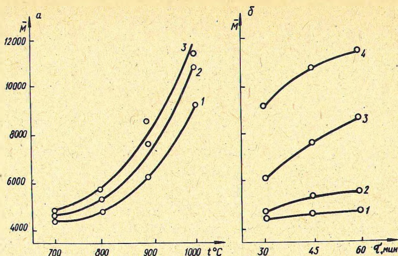
Рис. 1. Влияние температуры и продолжительности синтеза на молекулярный вес, \bar{M} стекловидных полифосфатов натрия, полученных из \text{NaH}_2\text{PO}_4 \cdot 2\text{H}_2\text{O} : а - 1 ÷ 3 - продолжительность синтеза 30, 45 и 60 мин, соответственно; б - 1 ÷ 4 - температура 700, 800, 900 и 1000 °С, соответственно.
