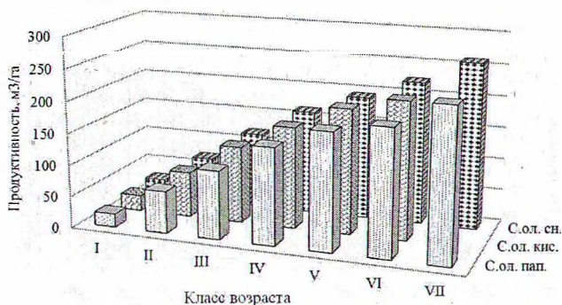
Рисунок 2 – Зависимость древесной продуктивности ( \text{м}^3/\text{га} ) сероольховых насаждений подзоны дубово-темнохвойных лесов от классов возраста в пределах наиболее распространенных типов леса
