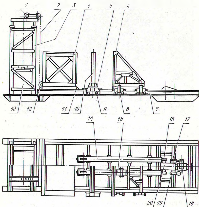
Рис. 2. Общий вид торцевыравнивающей установки ТГС 10.
