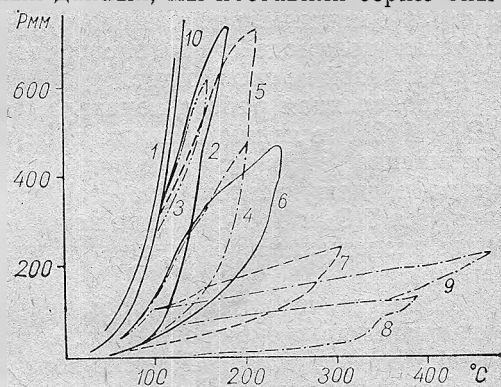
Рис. 4. Зависимость давления от температуры в системе с избытком \text{TiCl}_4 .
