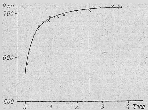
Рис. 2. Зависимость давления от продолжительности нагревания при t = 185^\circ .
