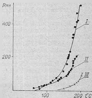
Рис. 3. Зависимость давления от температуры.
