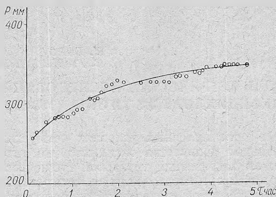
Рис. 1. Зависимость давления от продолжительности нагревания при t = 152^\circ .
